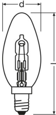
HAL PRO CL B 20 W 230 V E14, HAL CL B 28 W 230 V E14, HAL CL B 30 W 230 V E14, HAL PRO CL B 46 W 240 V E14
