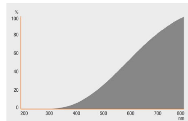
HAL PRO CL B 20 W 230 V E14, HAL PRO CL B 30 W 230 V E27, HAL PRO CL B 46 W 230 V E27, HAL PRO CL B 46 W 240 V E14
